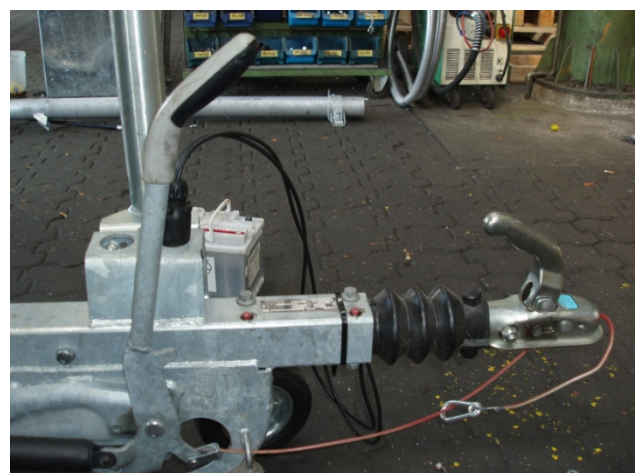
Levier du frein vers l'arrière = frein desserré
