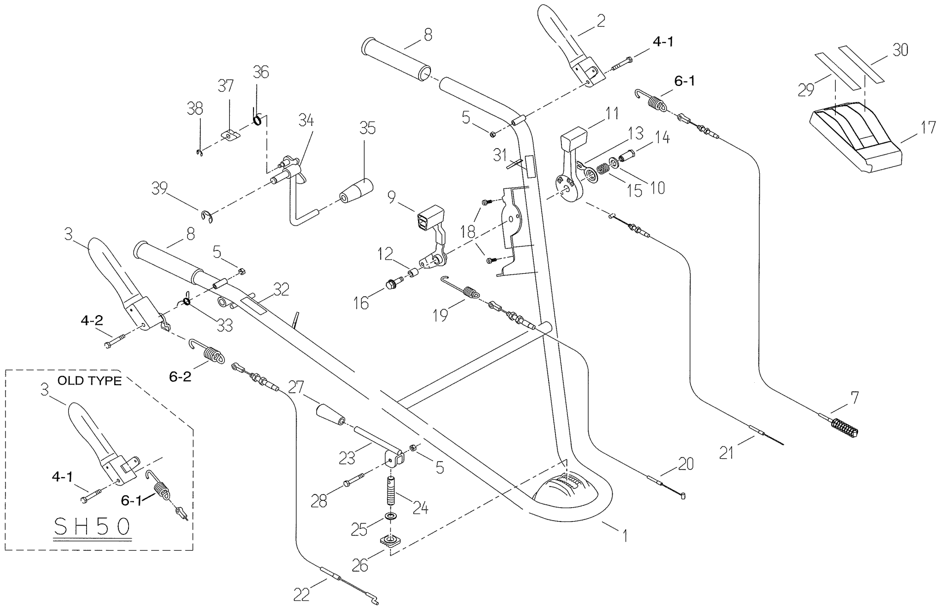
Fig. 1 HANDLE
