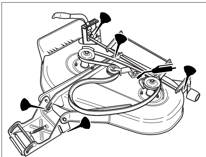
Figure 10. Points de lubrification de la tondeuse
