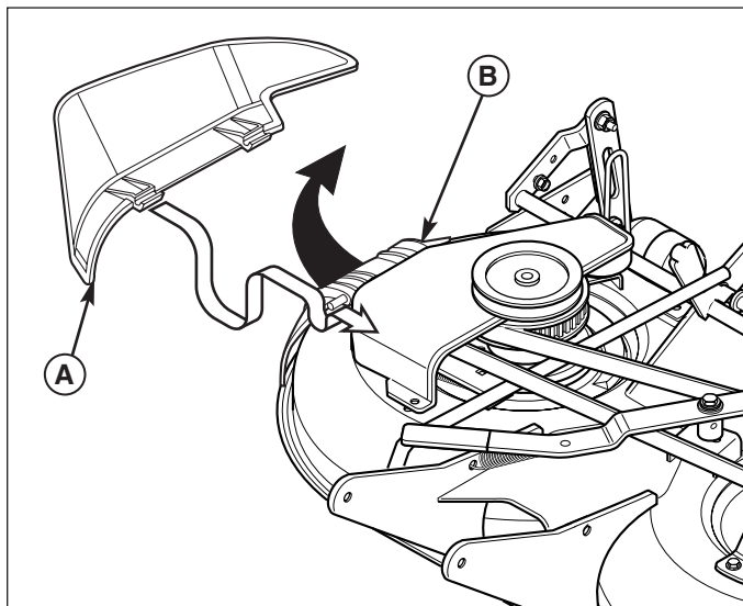
Figure 3. Installation du déflecteur d'éjection latérale
