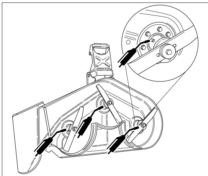
Figure 12. Points de lubrification d'arbre moteur
