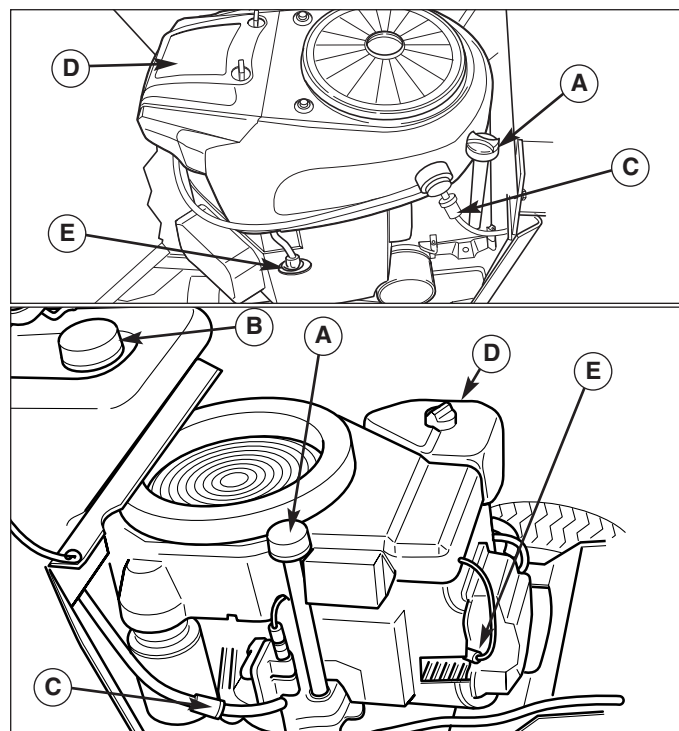
Figure 9. Compartiment moteur
