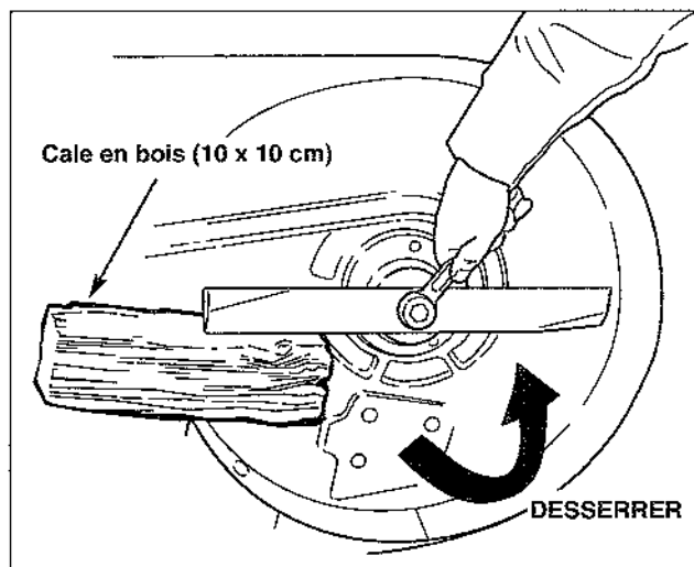
Figure 22. Dépose de la lame
