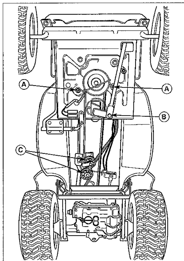
Figure 41. Remplacement de la courroie de transmission
