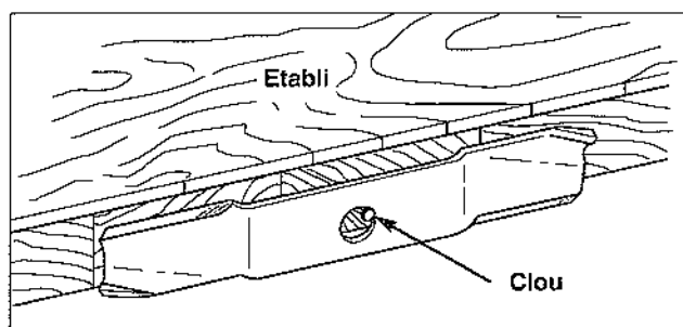
Figure 23. Equilibrage de la lame
