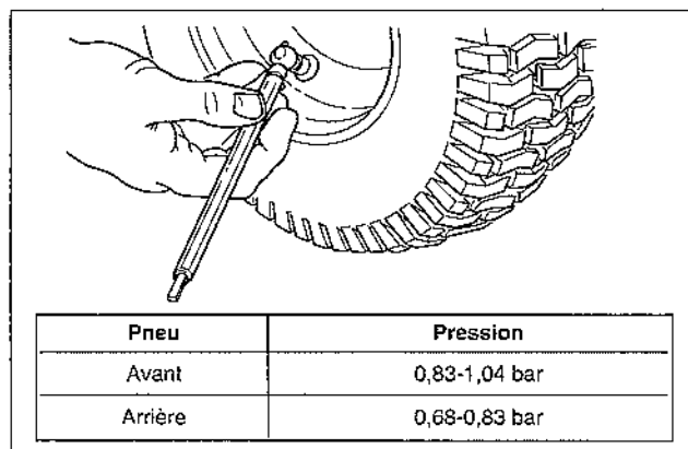
Figure 11. Vérification de la pression des pneus
