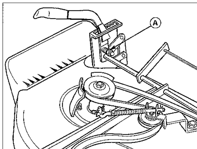
Figure 37. Réglage de la tension de la poignée
