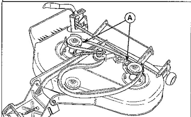
Figure 13. Embrayage et système de frein de la tondeuse
