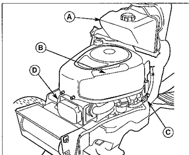
Figure 10. Compartiment moteur
