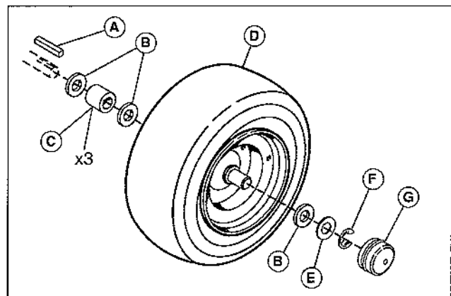
Figure 21. Lubrifier les arbres d'essieu arrière
