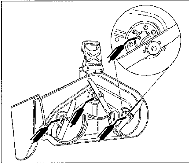
Figure 19. Points de lubrification des arbres
