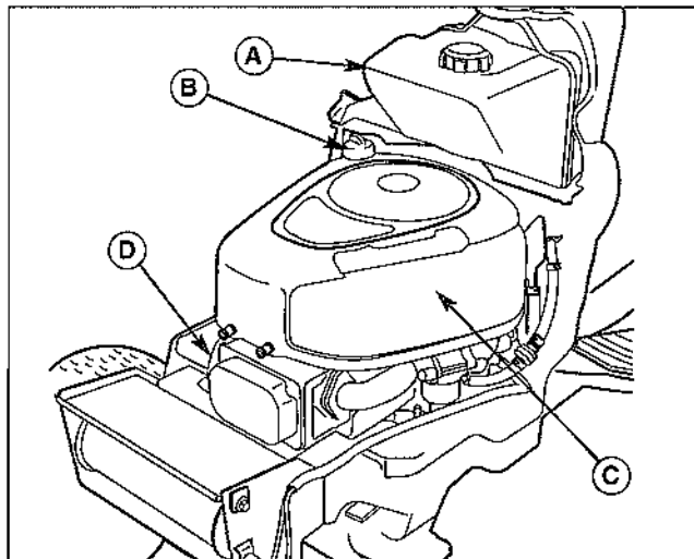
Figure 12. Compartiment moteur
