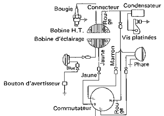
SCHEMA DE CABLAGE
