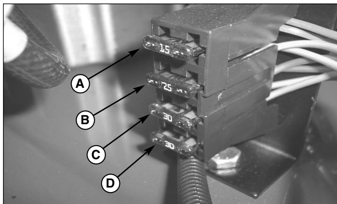
Figure 37. Désignation et calibres des fusibles
