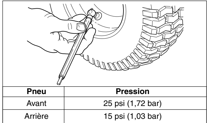
Figure 17. Vérification de la pression des pneus
