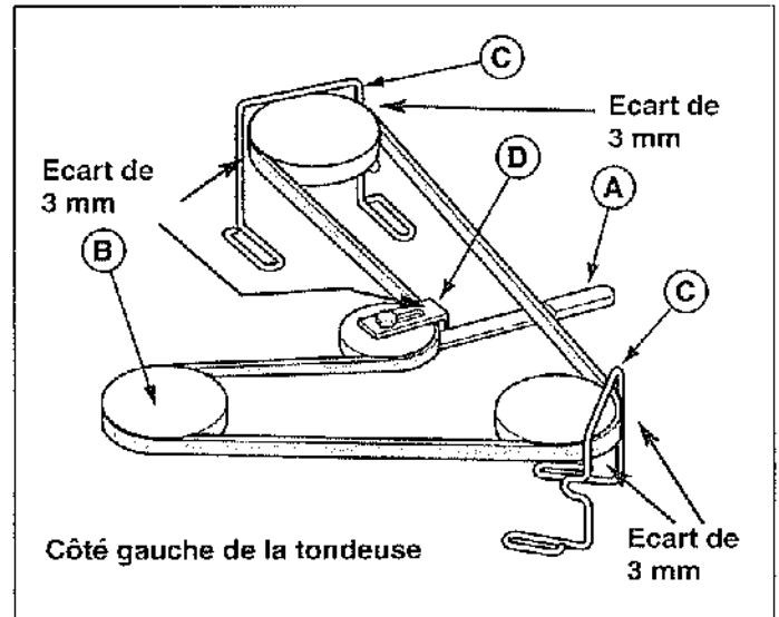
Figure 69. Acheminement de la courroie de tondeuse – Tondeuse de 97 cm
