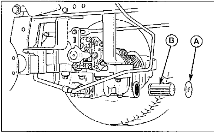
Figure 44. Entretien du filtre de transmission interne A. Bouchon d'accès au filtre B. Filtre interne
