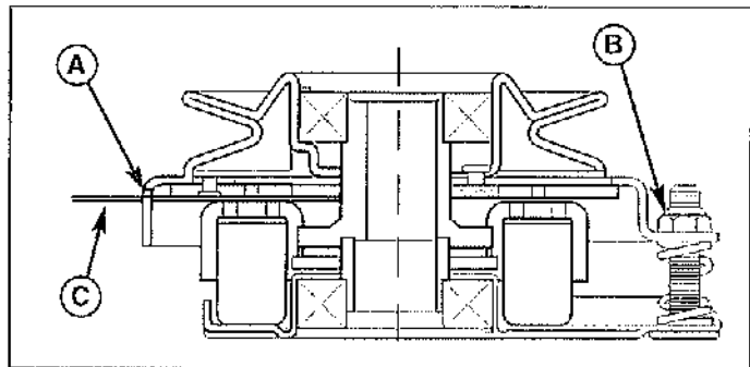
Figure 53. Réglage de l'embrayage de la PDF A. Orifice de réglage B. Ecrou de réglage C. Jauge d'épaisseur
