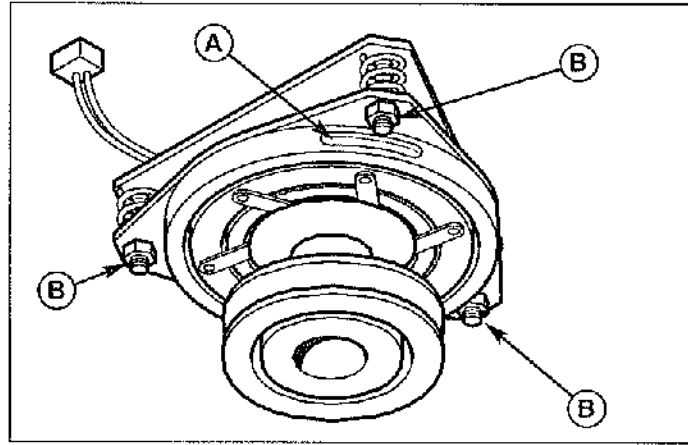
Figure 52. Réglage de l'embrayage de la PDF A. Orifice de réglage (quantité 3, une illustrée) B. Ecrou de réglage
