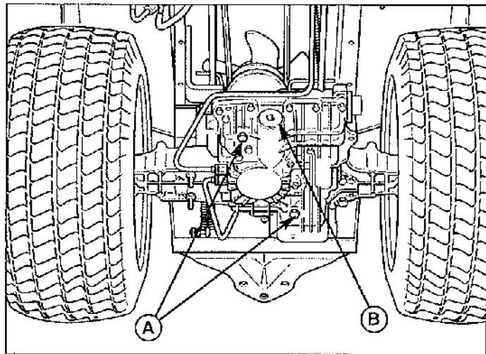
Figure 45. Bouchons de vidange de transmission A. Bouchons de vidange de 14 mm B. Bouchon d'accès au filtre
