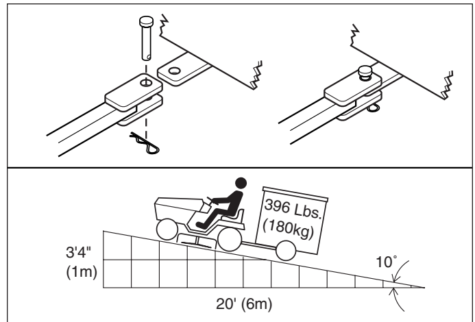
Figure 20. Recommandations de poids de remorque
