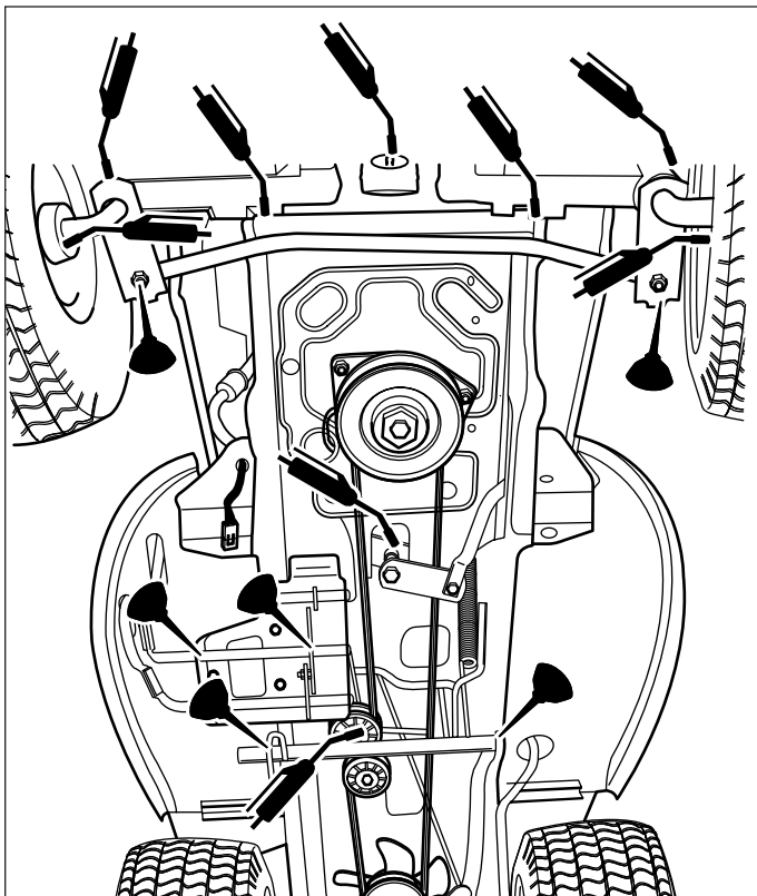
Figure 26. Lubrification du tracteur
