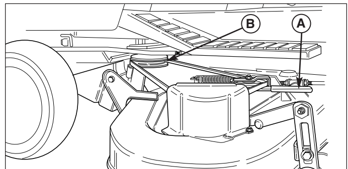
Figure 11. Dépose et installation de la courroie
