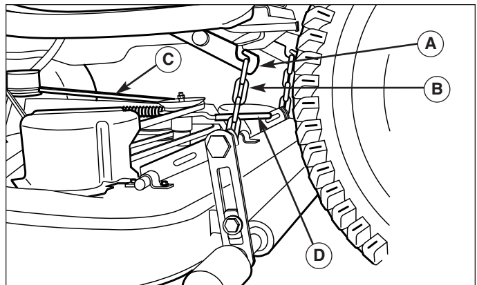
Figure 16. Relevage de tondeuse
