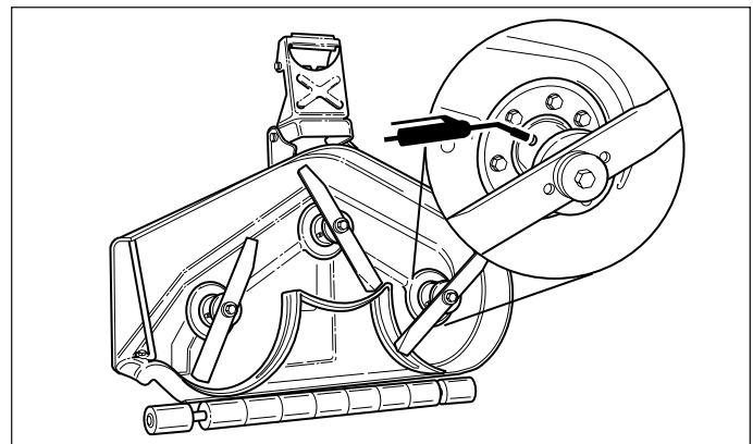
Figure 29. Points de lubrification d'arbre moteur
