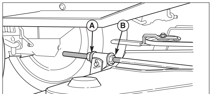
Figure 60. Mise à niveau longitudinale de la tondeuse
