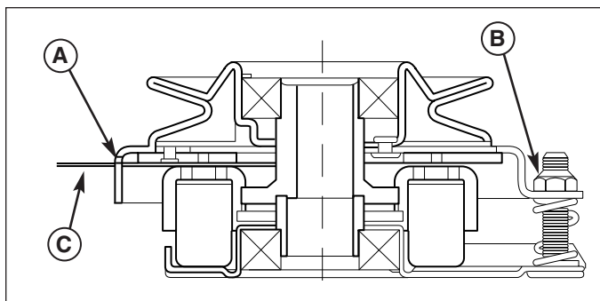
Figure 53. Réglage de l'embrayage de la PDF
