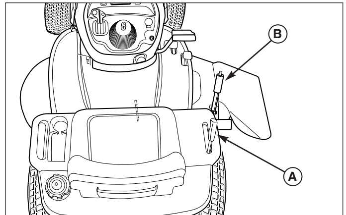
Figure 7. Relevage et abaissement de la tondeuse (Modèles de 102 cm)
