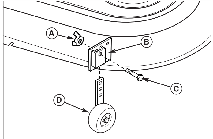
Figure 55. Réglage de la roue d'ajustement à glissement
