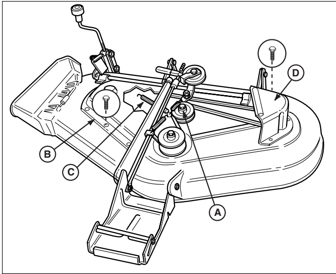
Figure 63. Tondeuse - Modèles de 112 et 127 cm
