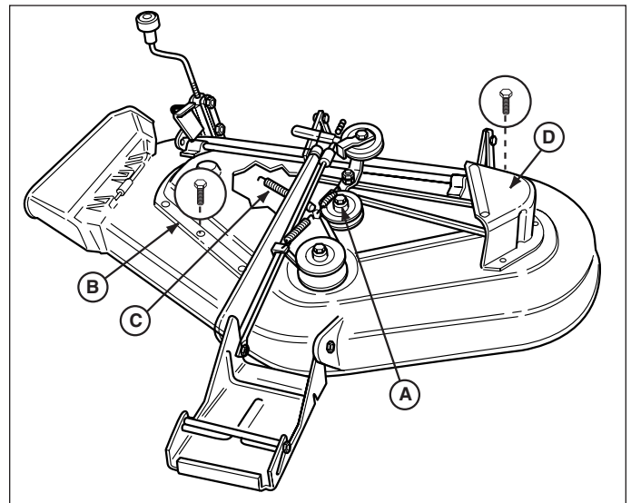
Figure 62. Tondeuse - Modèles de 112 et 127 cm
