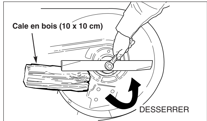
Figure 32. Dépose de la lame
