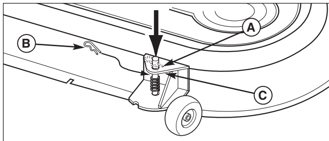
Figure 54. Réglage des roulettes-guides
