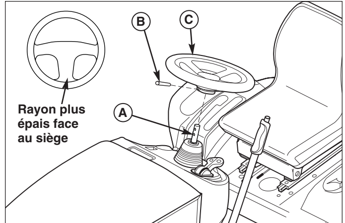
Figure 49. Composants du volant
