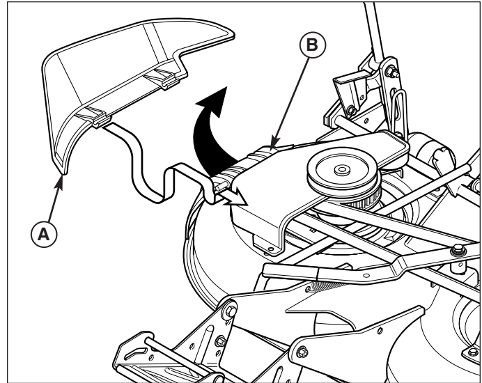
Figure 5. Installation du déflecteur d'éjection latérale
