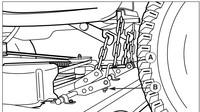
Figure 59. Mise à niveau latérale de la tondeuse - Modèles de crochets en forme de J
