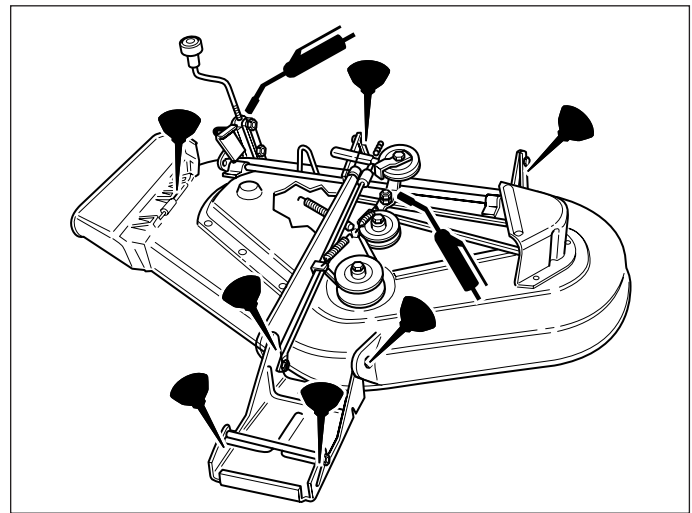
Figure 28. Points de lubrification de la tondeuse
