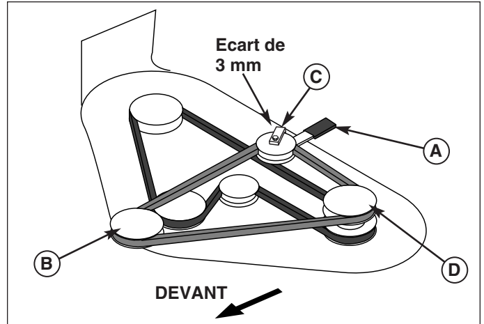
Figure 61. Acheminement de la courroie de tondeuse
