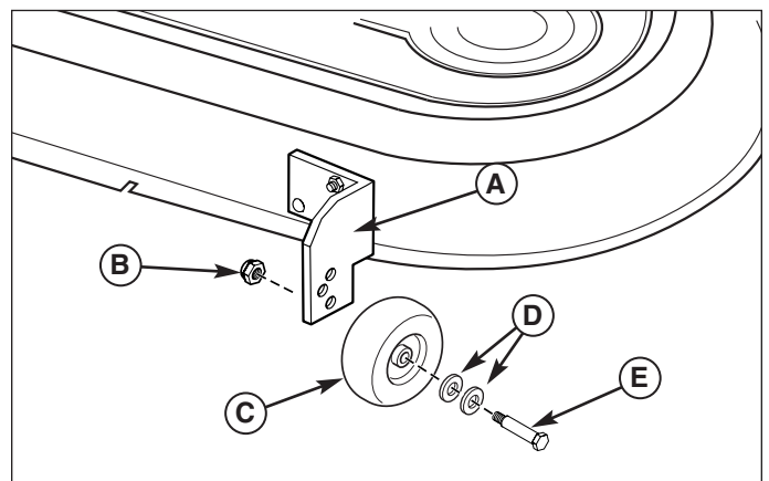
Figure 56. Réglage des roues d'ajustement à support fixe
