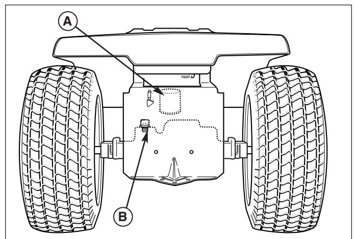
Figure 43. Filtre d'huile de circuit hydraulique
