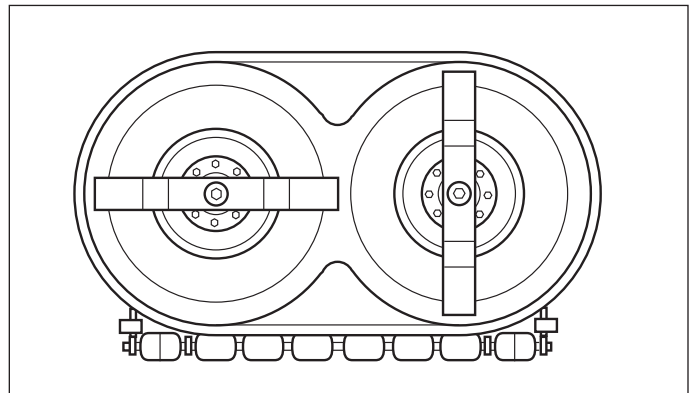
Figure 69. Synchronisation des lames de tondeuse
