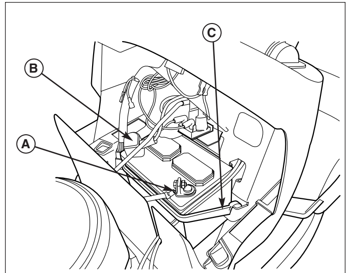
Figure 25. Batterie
