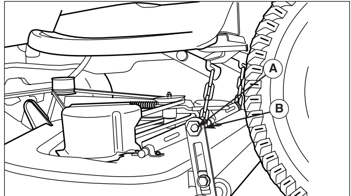
Figure 58. Mise à niveau latérale de la tondeuse - Modèles d'écrous excentriques
