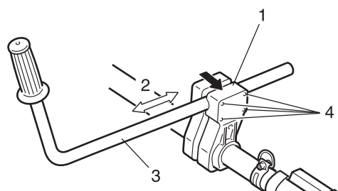
1. Support de poignée 3. Poignée gauche 2. Réglage 4. Boulon M5×35
