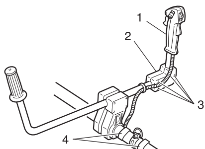
1. Poignée droite 3. Boulon M5×25 2. Support 4. Collier de fixation du câble
