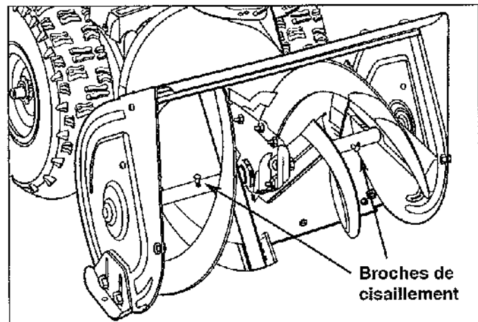
Figure 31. Remplacement des broches de cisaillement
