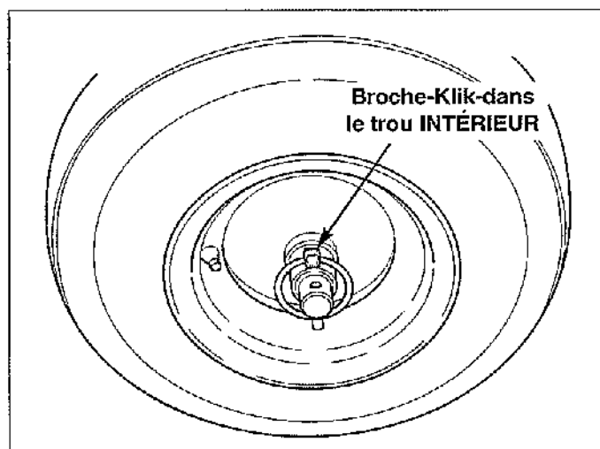
Figure 12. Blocage de l'entraînement de traction - Engagé
