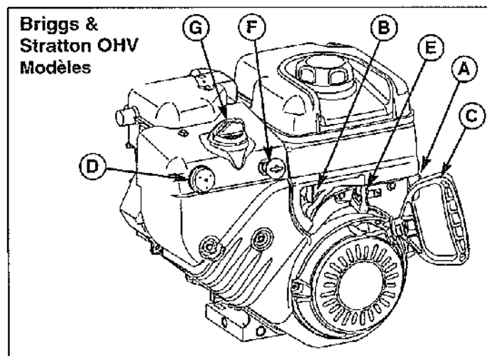
Figure 2. Commandes du moteur
