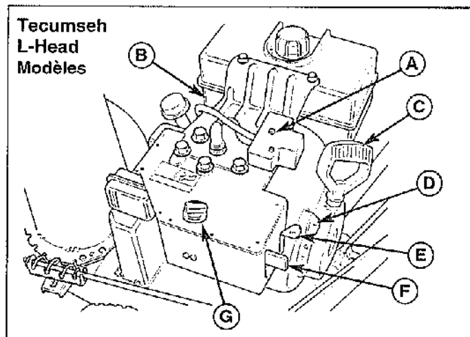
Figure 5. Commandes du moteur
