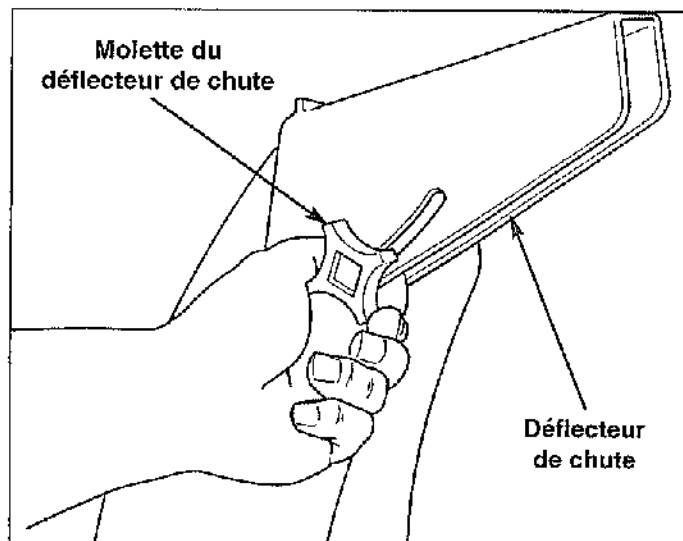
Figure 9. Réglage du déflecteur de chute
