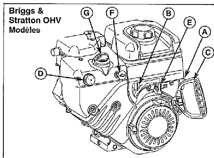
Figure 6. Commandes du moteur
