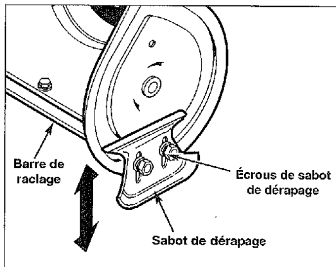
Figure 10. Réglage des sabots de dérapage
