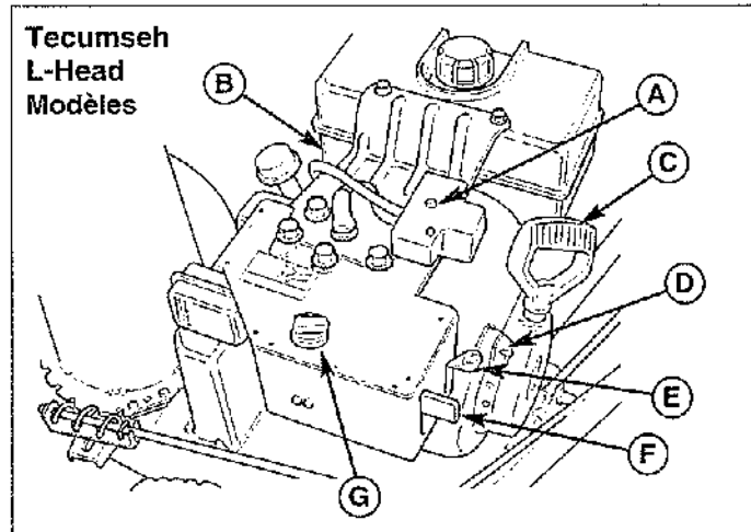
Figure 1 Commandes du moteur
