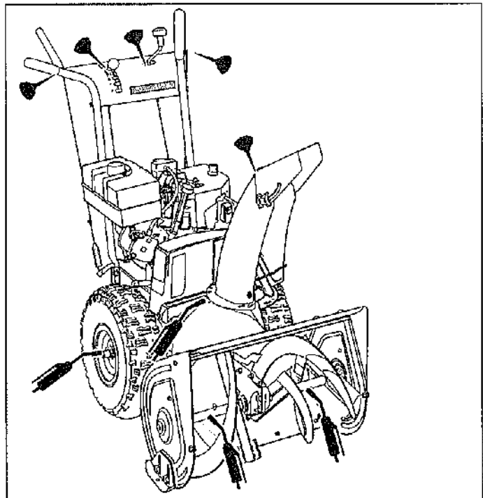
Figure 16. Principaux points de lubrification du chasse-neige
